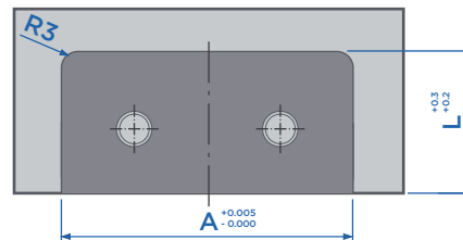
Placas Porta Macho/Fêmea
